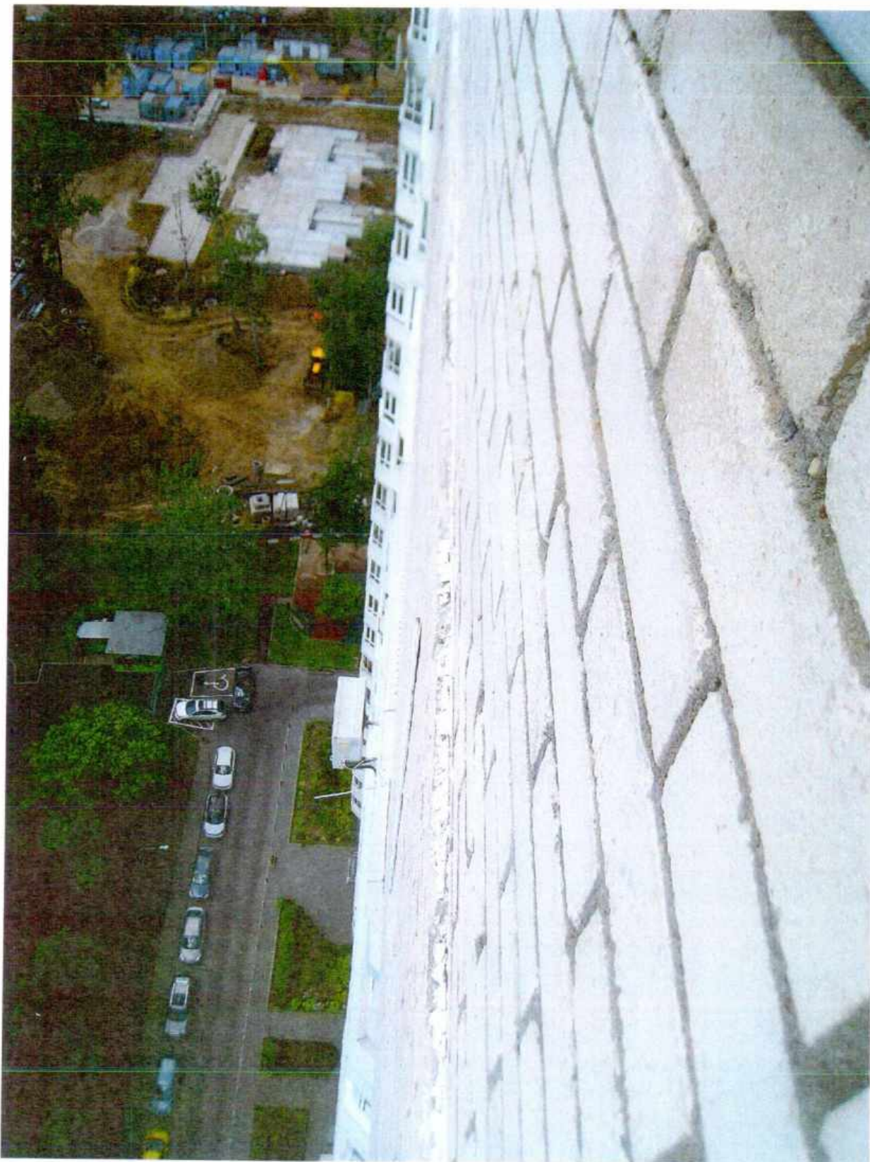
Фото 10. В уровне перекрытия над техническим этажом в габаритах части помещений №№11,12,13,18 (смотри план БТИ) смещение плоскости парапета крыши вовнутрь до 40мм
