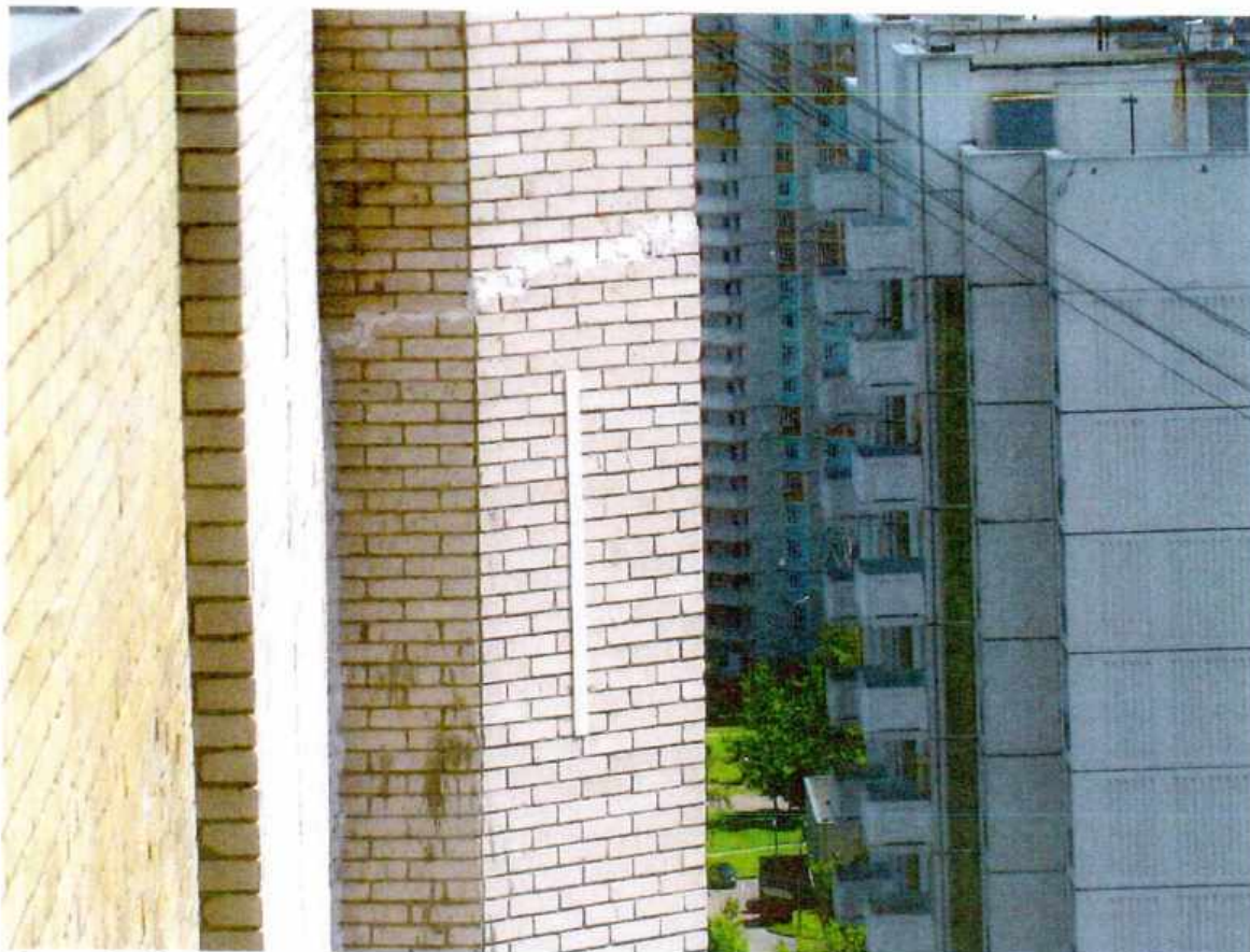
Фото 6. Отклонение плоскости наружной стены со стороны фасада в габаритах части помещений №№11,12,13,18 (смотри план БТИ) в уровне технического этажа от вертикали наружу с увеличением отклонения в верхней части, в уровне перекрытия над техническим этажом имеется смещение плоскости парапета крыши вовнутрь до 40мм
